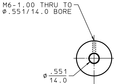
DRIVE CPLG BORE DETAIL 71
