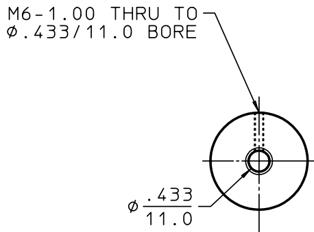
DRIVE CPLG BORE DETAIL 63
